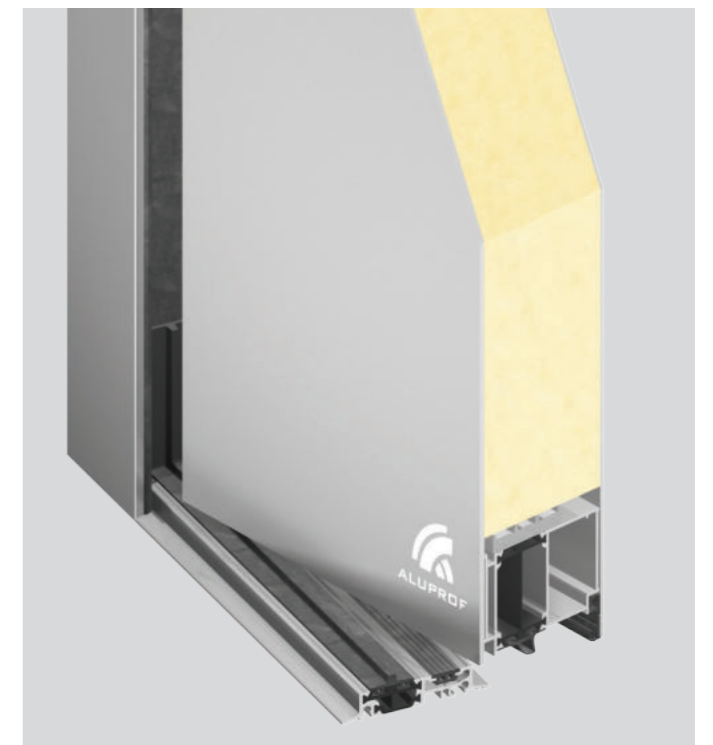
ALUPROF MB 86
