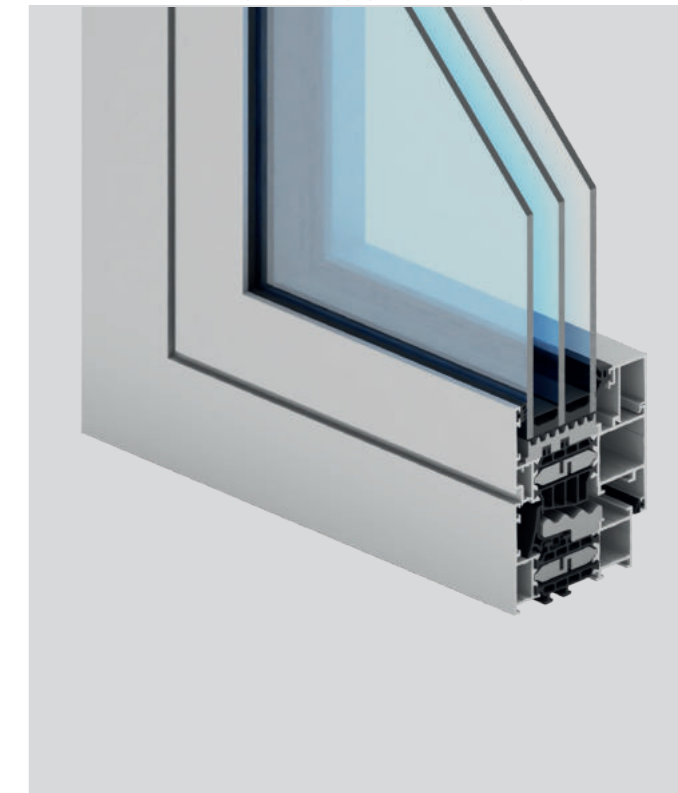
ALIPLAST GENESIS 90 OKNO Z WYSOKĄ IZOLACJĄ TERMICZNĄ
