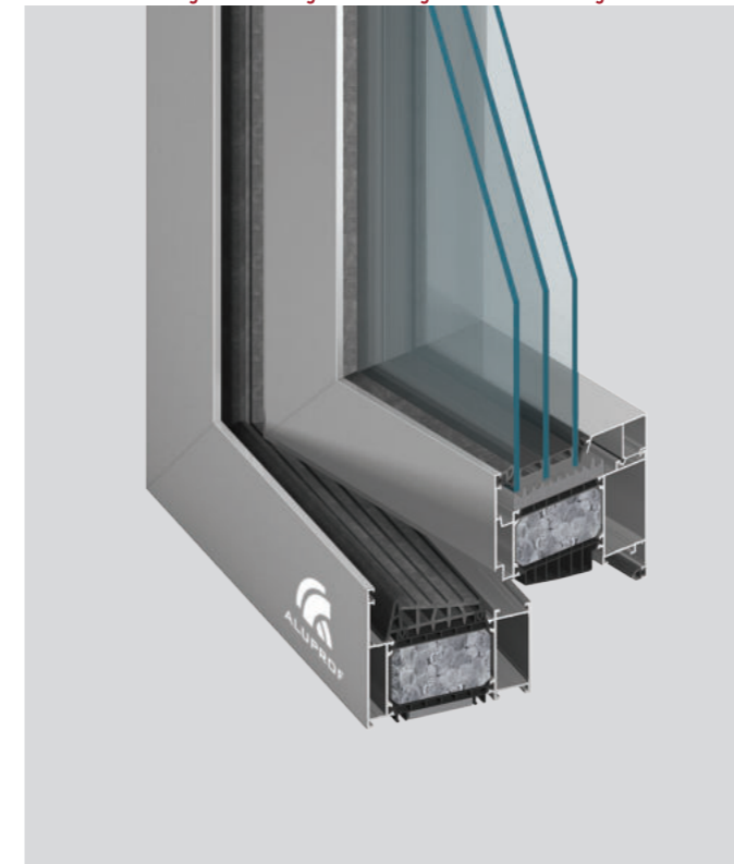
ALUPROF MB 104 PASSIVE OKNO O NAJWYŻSZEJ IZOLACJI TERMICZNEJ
